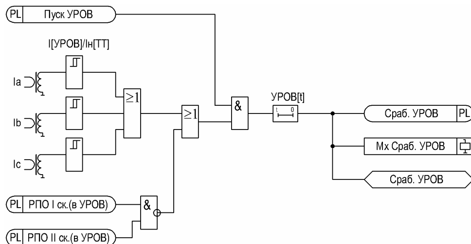
Рисунок 11 – Функциональная схема алгоритма УРОВ.
