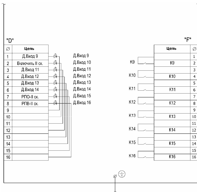
Рисунок А.2 - Подключение внешних цепей к блоку DMV-EP-02 (окончание)
