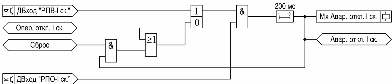
Рисунок 16 – Функциональная схема алгоритма аварийной сигнализации.
