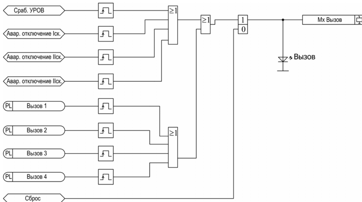
Рисунок 15 – Функциональная схема алгоритма вызывной сигнализации.
