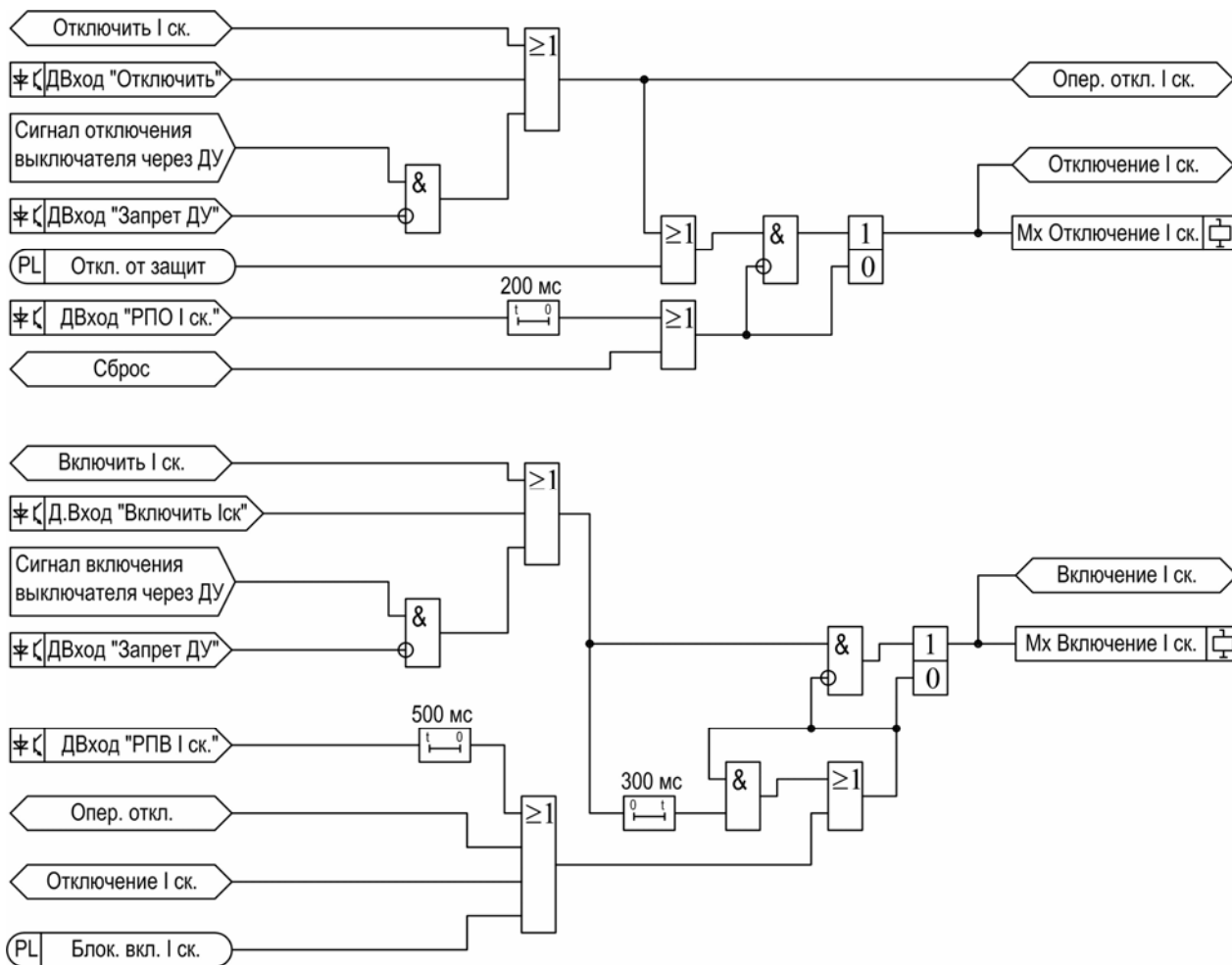
Рисунок 14 – Функциональная схема алгоритма управления выключателем.
