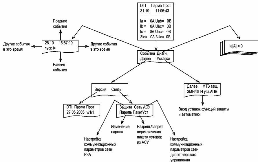
Рисунок 16 – Структура меню блока DMV-SP
